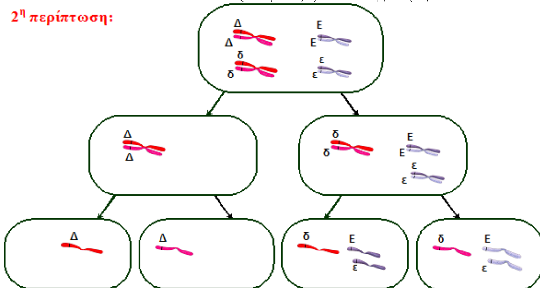
Εικόνα 2: Μη διαχωρισμός ομολόγων χρωμοσώματων κατά την πρώτη μειωτική διαίρεση. Οι γαμέτες που προκύπτουν έχουν γονιδιακή σύσταση Δ_, δΕε.
